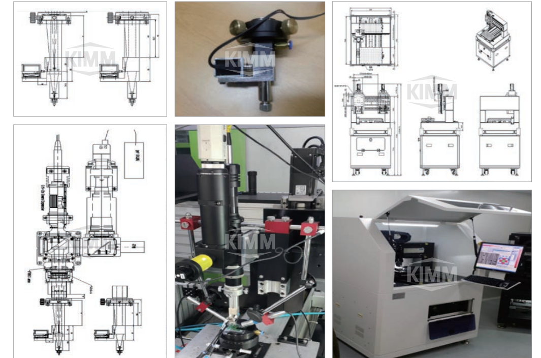
< 레이저 솔더링 광학계 및 시스템 >
