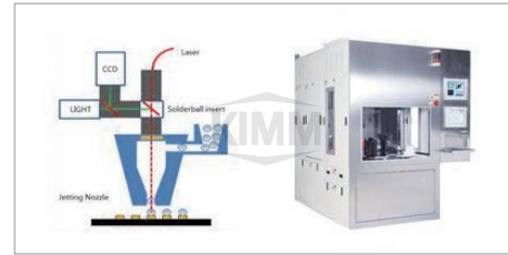
< 레이저 솔더링 헤드 및 시스템 >
